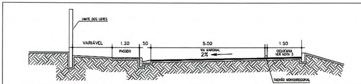
Figura 5 – Seção transversal tipo das vias marginais.
