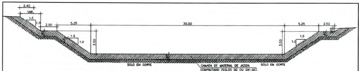
Figura 2 - Seção transversal tipo do canal do Igarapé Ilha do Coco.
