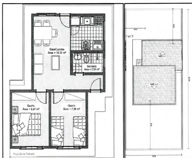
Figura 7 – Planta baixa e de cobertura da Unidade Habitacional Tipo.
